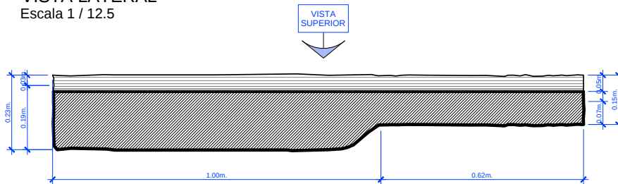
SECCION LONGITUDINAL Escala 1 / 12.5
