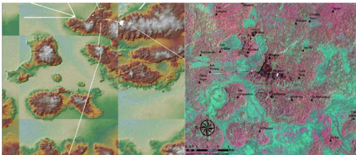
Fig. 16: Huellas fósiles en la escala regional de la Cuenca Mirador (FARES, 2012)
